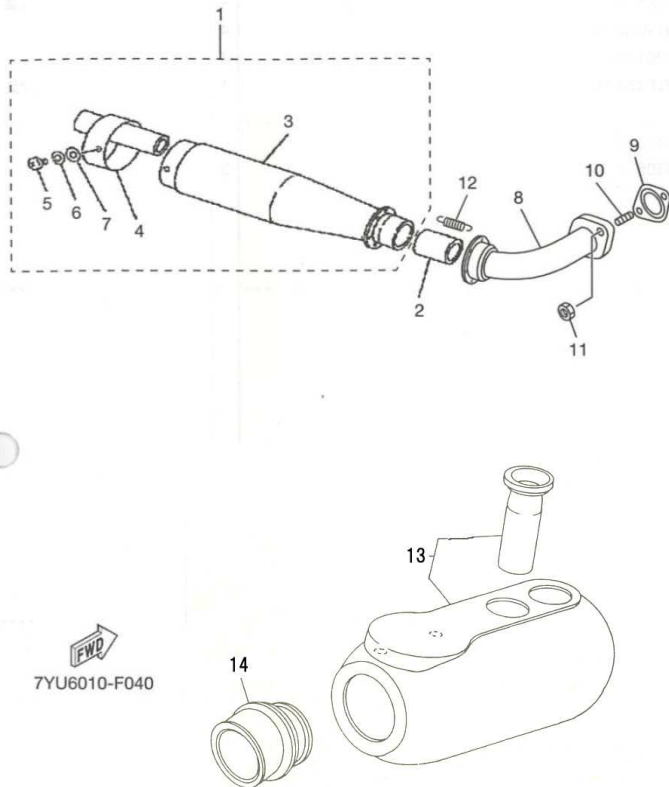
FIG. 4 エキゾースト
